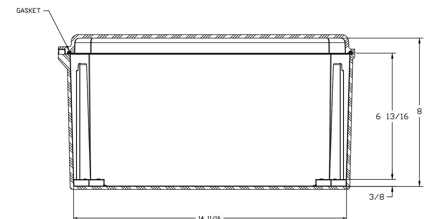
SECTION A-A
