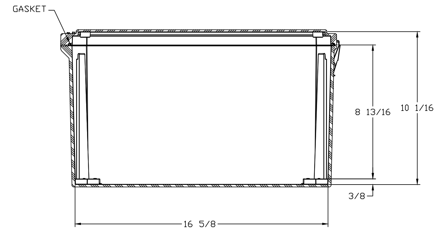
SECTION A-A
