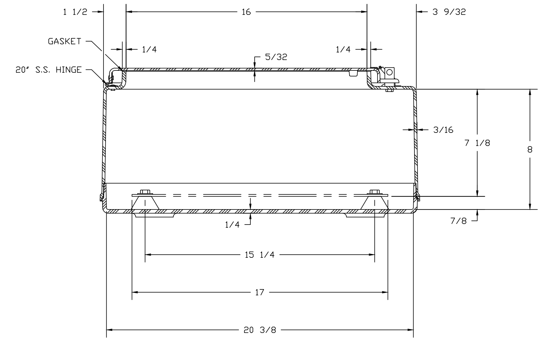
SECTION A-A
