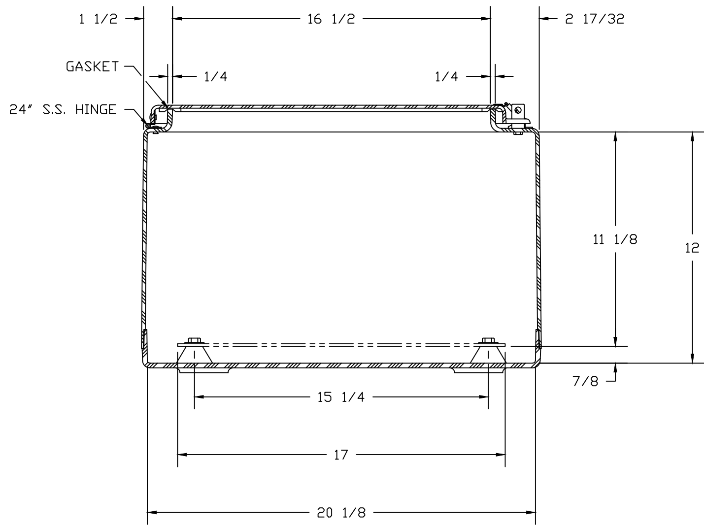
SECTION A-A
