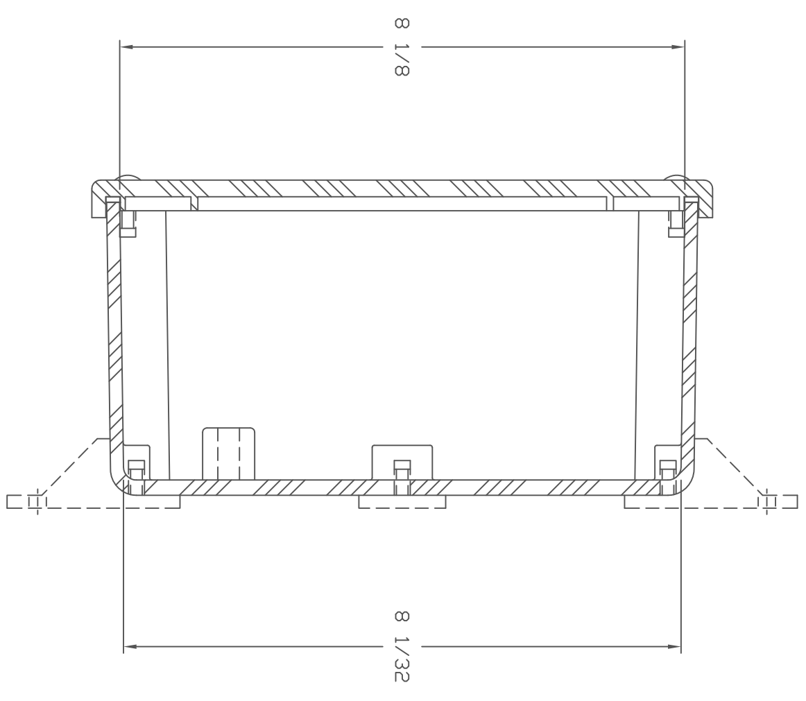
SECTION A-A
