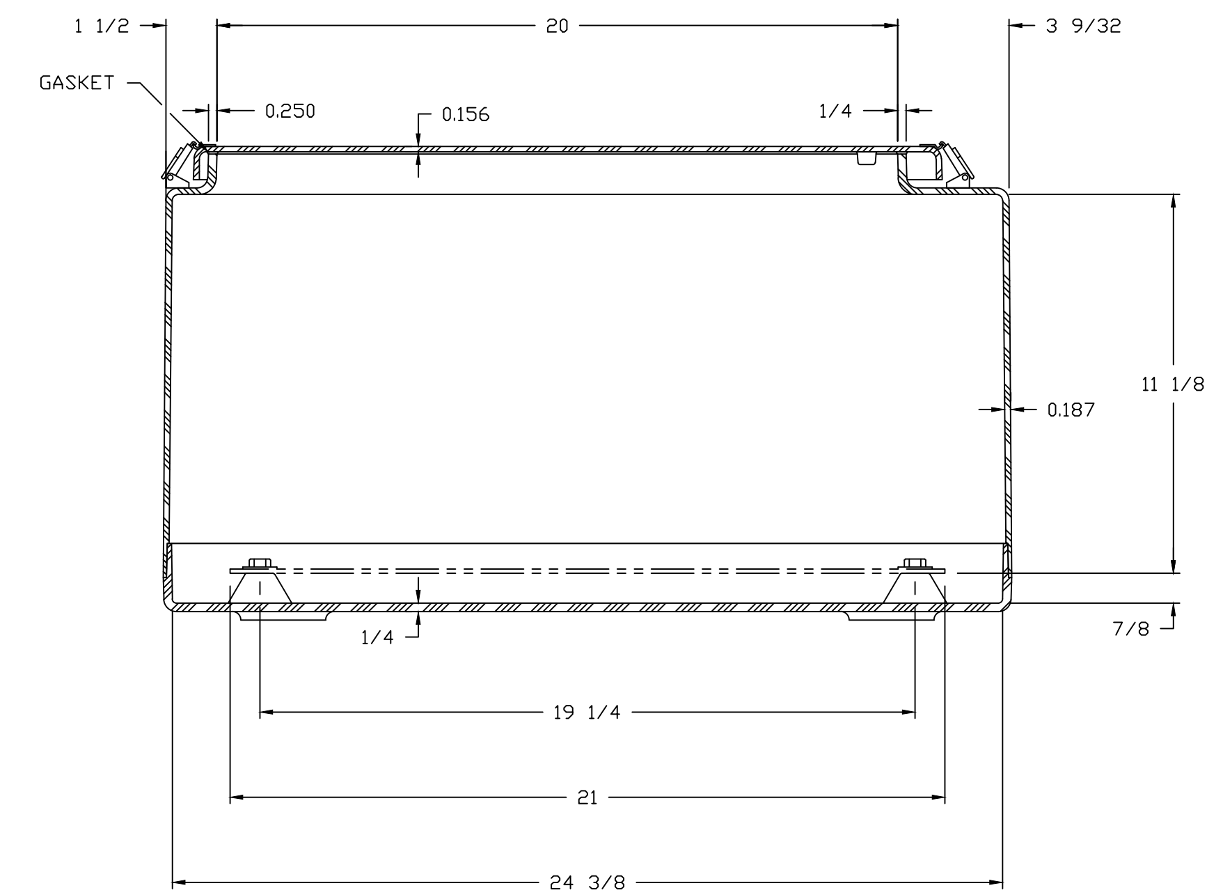
SECTION A-A
