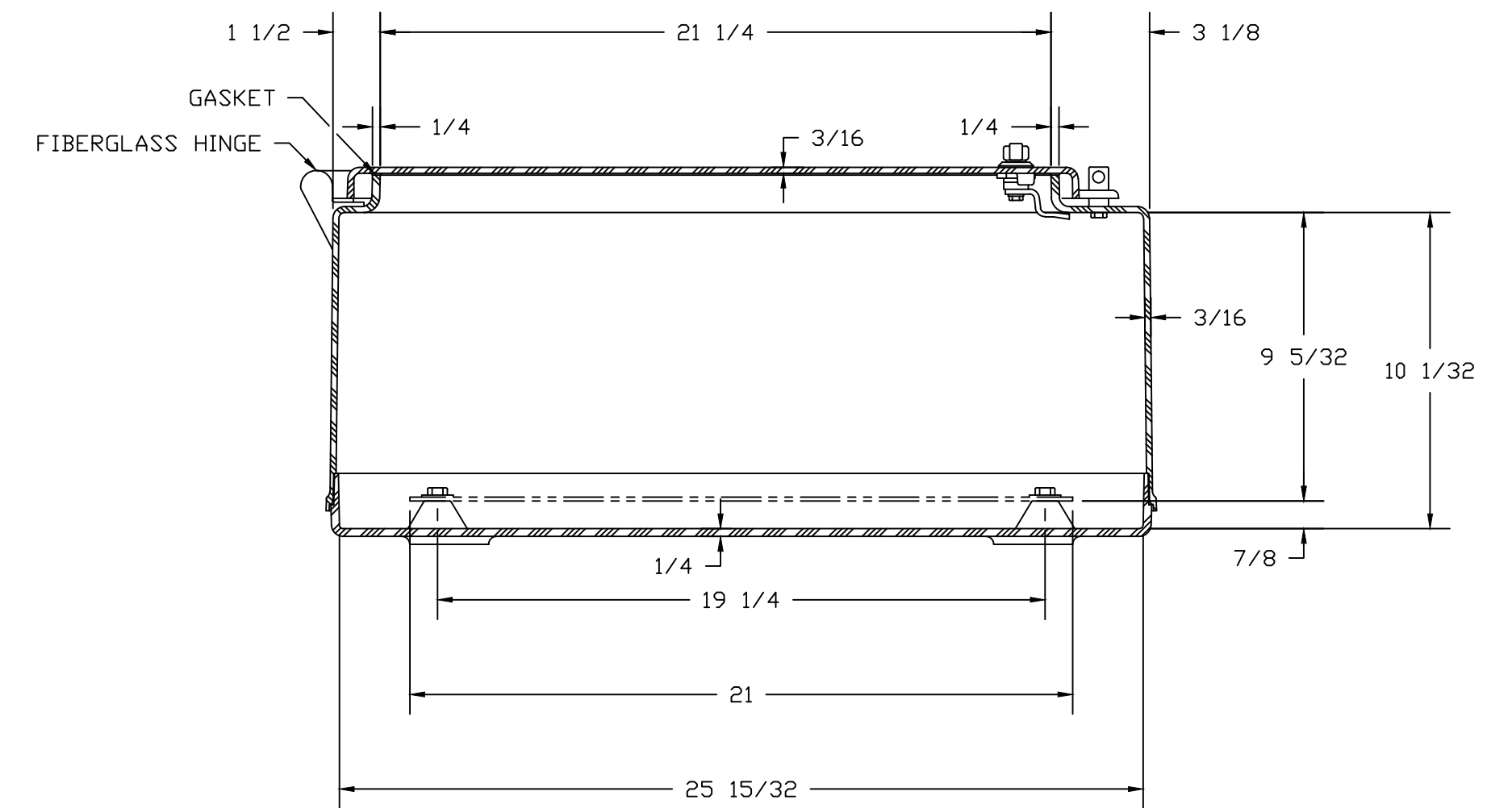
SECTION A-A
