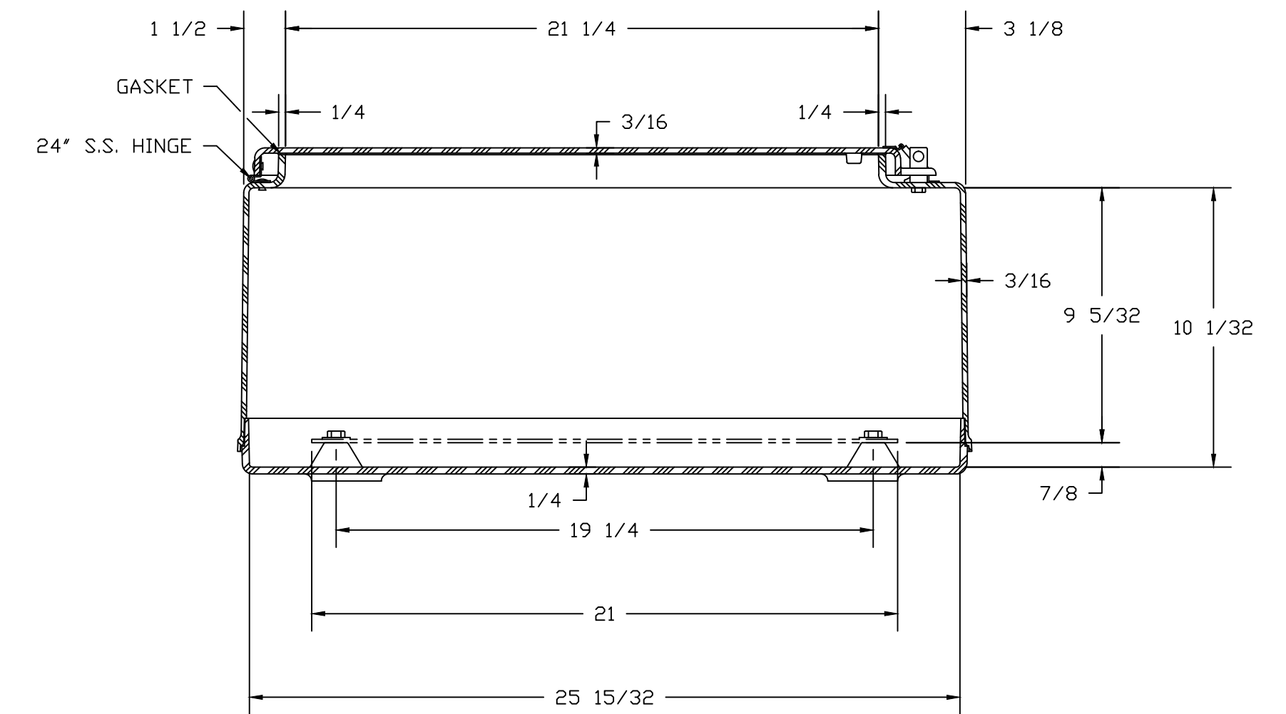
SECTION A-A
