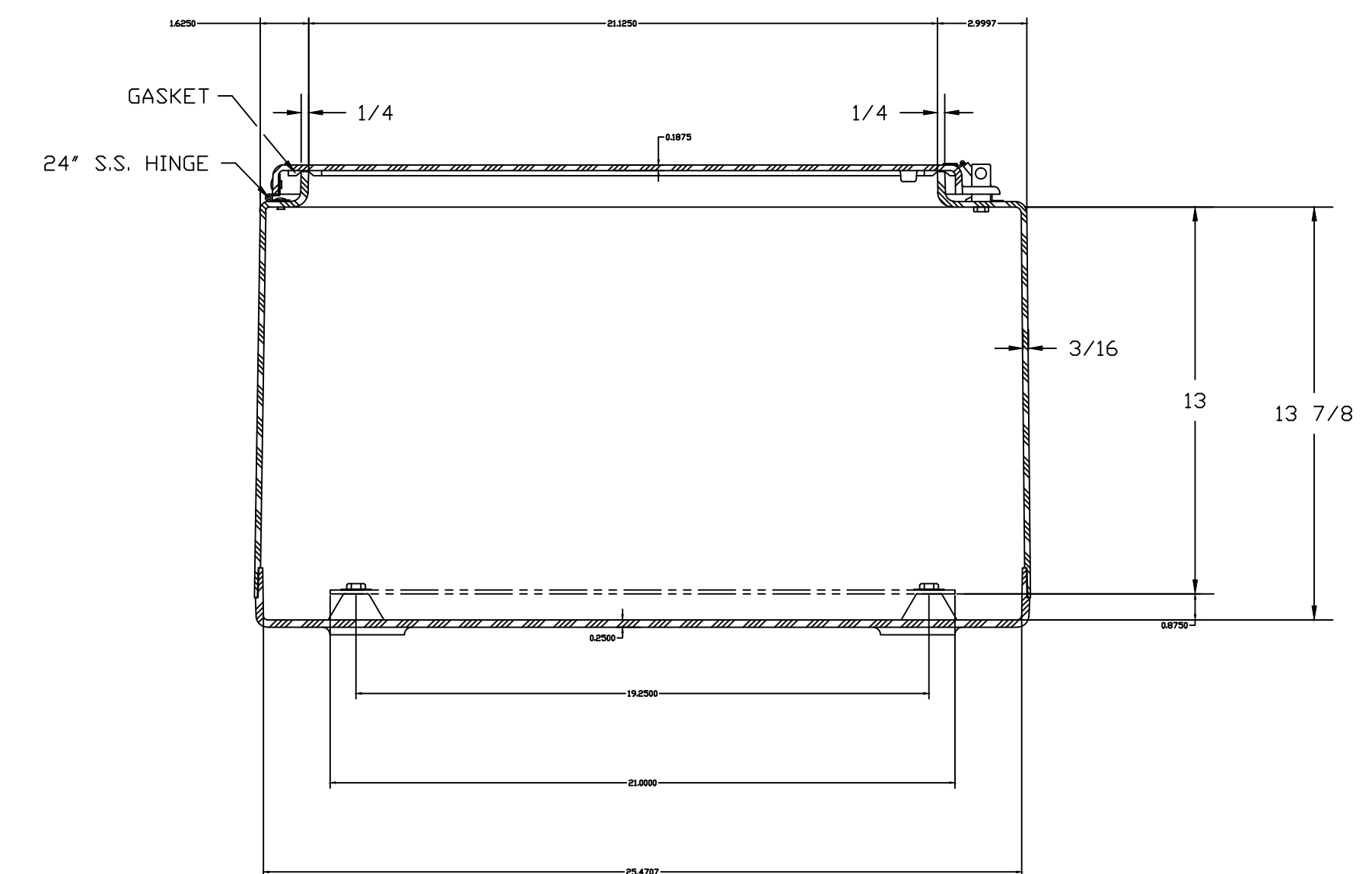
SECTION A-A
