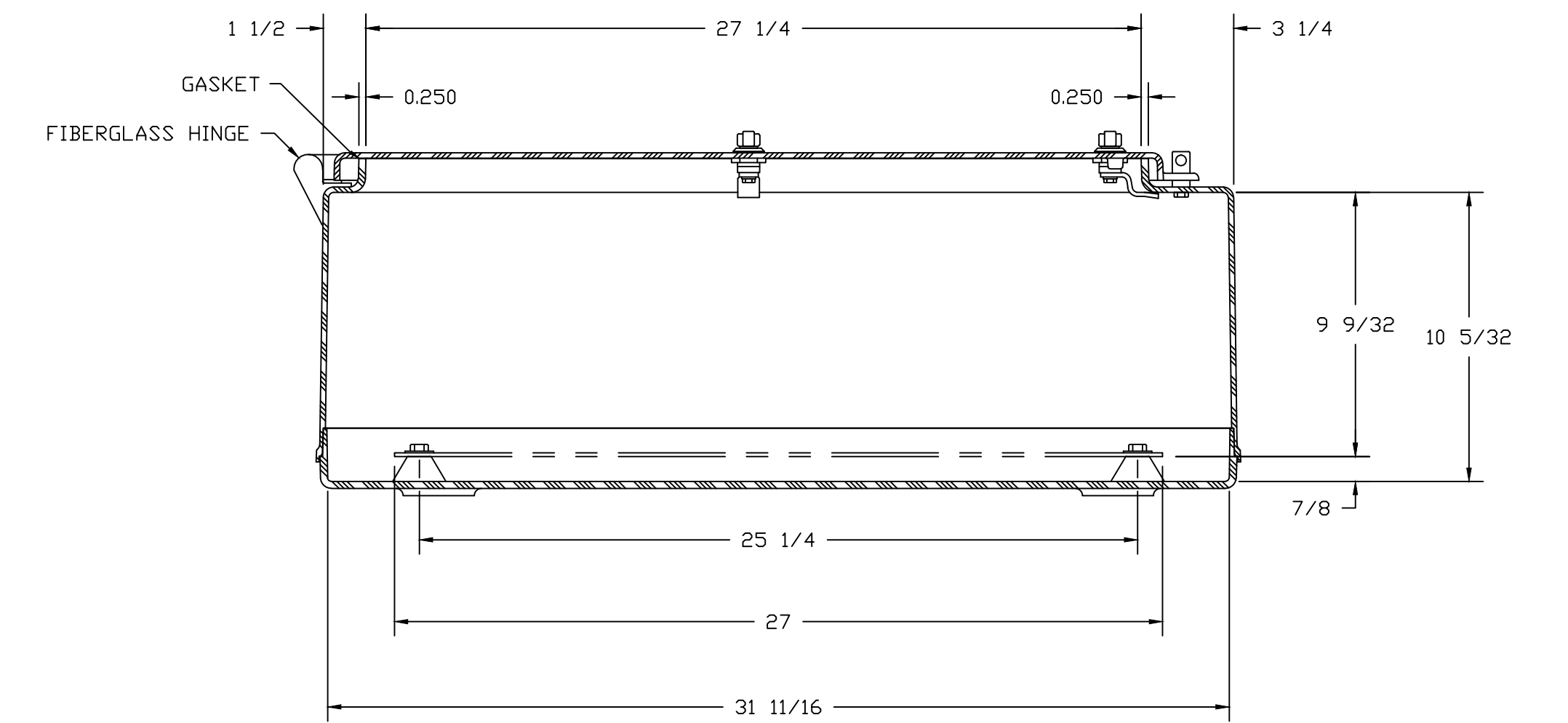
SECTION A-A
